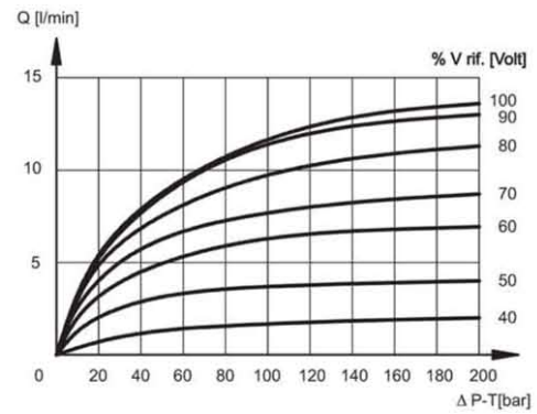
SPOOL TYPE A04
