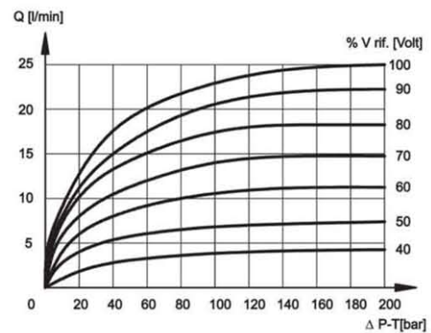
SPOOL TYPE A08
