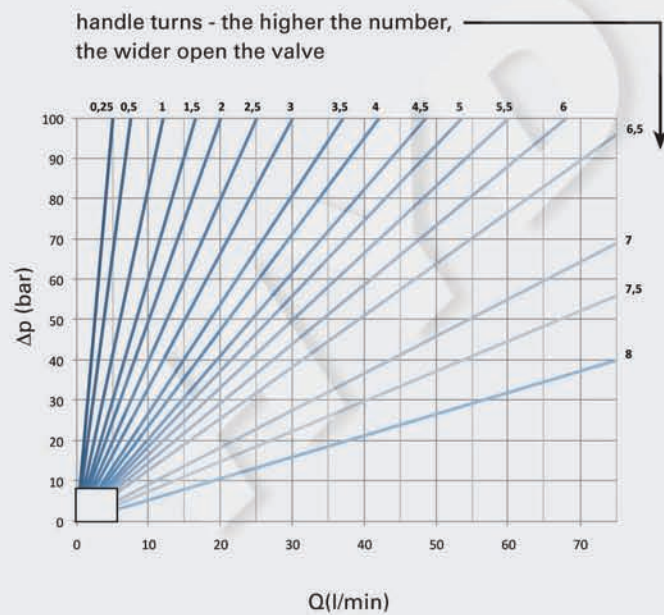
NDV/NDRV/NDVP/NDRVP-DN10
