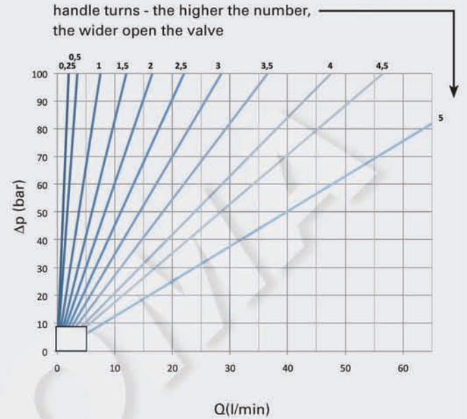
NDV/NDRV/NDVP/NDRVP-DN12
