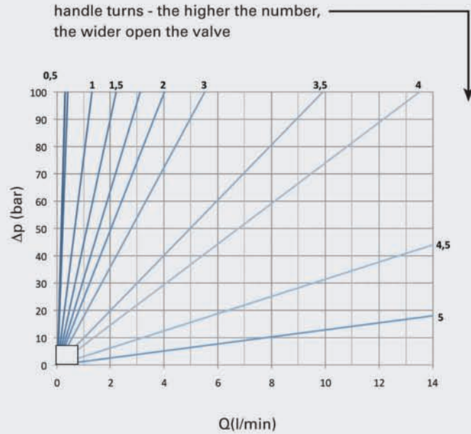
NDV/NDRV/NDVP/NDRVP-DN10
