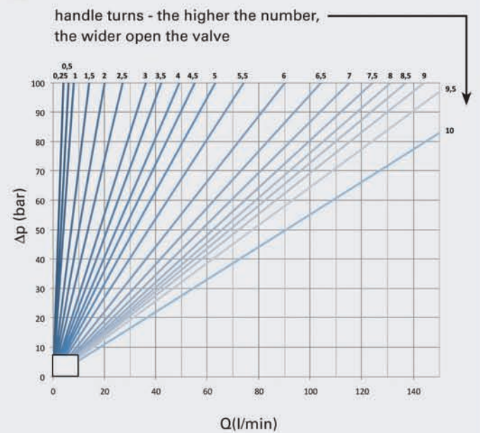
NDV/NDRV/NDVP/NDRVP-DN12
