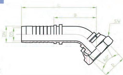
Koleno 45° Elbow 45°
