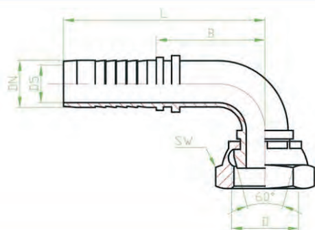
Koleno 90° Elbow 90°
